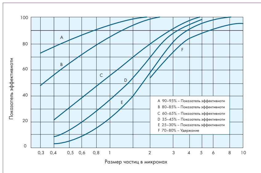
■ Рис. 8. Типичные показатели эффективности воздушных фильтров по отношению к размерам твердых частиц. Используются данные Американского общества инженеров по отоплению, охлаждению и кондиционированию воздуха (ASHRAE)
